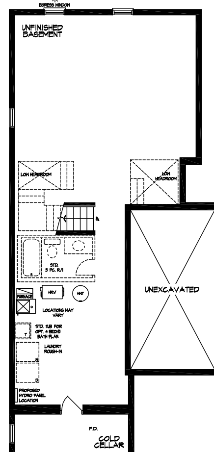
BASEMENT ELEVATION A1, A2 (REV), B1 & B2 (REV)
